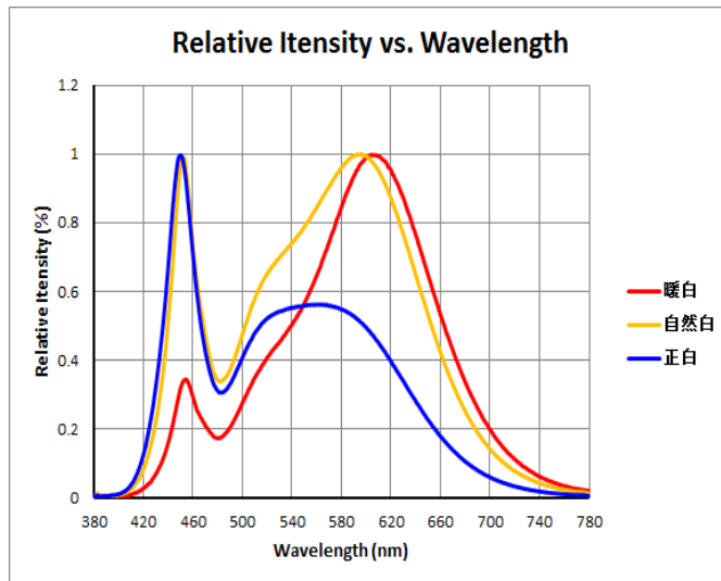
Spectrum Distribution (IF = 150 mA, Ts = 25 °C) 光谱分布图
